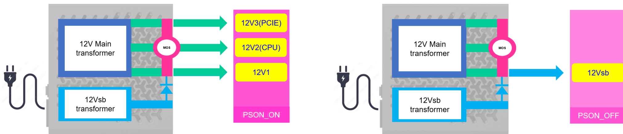
Inte 12VO V03 Main Power Connector Pin-Out
